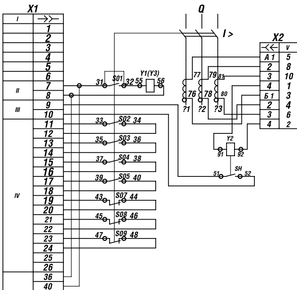
Рисунок Б.1 Схема электрическая принципиальная выключателя Э06 переменного тока с ручным приводом.
